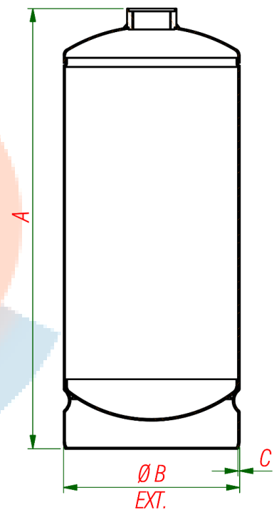
Figura 2 - Recipiente para Agente Extintor
