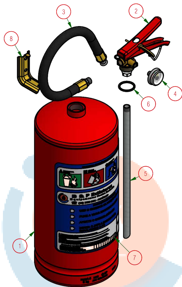
Figura 1 - Componentes do Extintor de Incêndio 8 kg ABC
