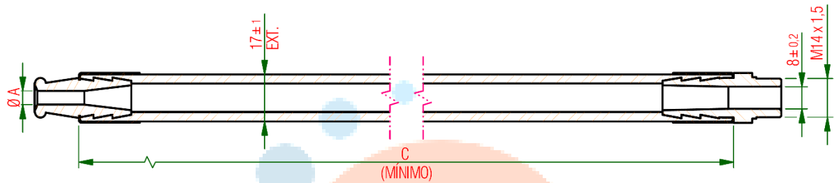
Figura 4 - Dimensões da Mangueira de Descarga
