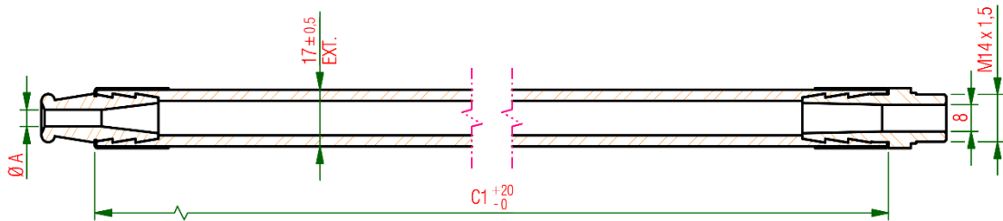
Figura 4 - Dimensões da Mangueira de Descarga
