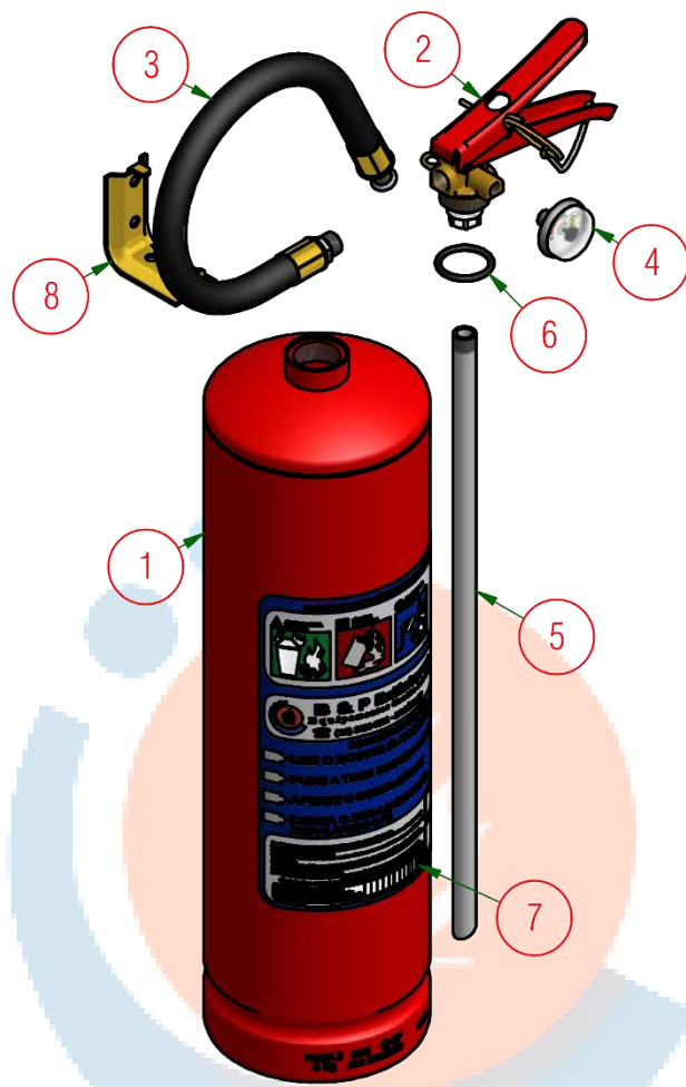
Figura 1 - Componentes do Extintor de Incêndio 6 kg ABC
