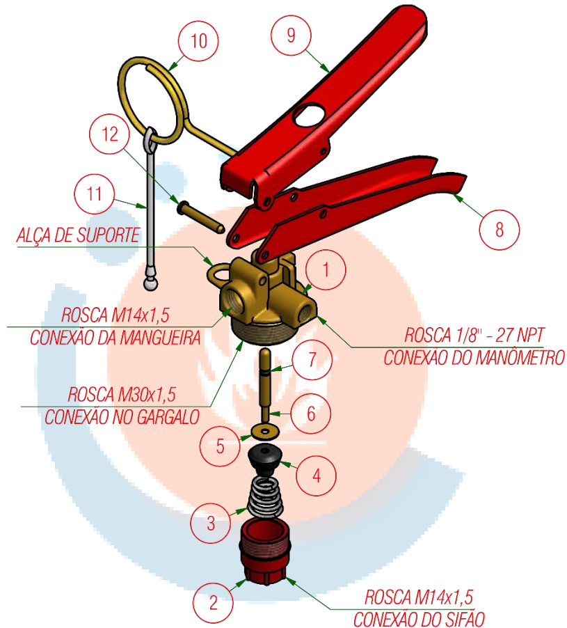
Figura 3 - Componentes da Válvula de Descarga dos Extintores de Pó Químico
