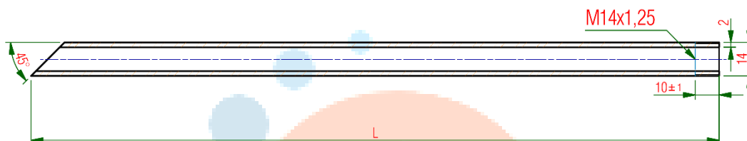
Figura 7 - Dimensões do Tubo Sifão
