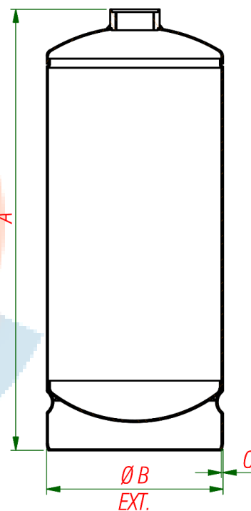
Figura 2 - Recipiente para Agente Extintor
